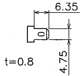
端子部詳細 (1:1)
